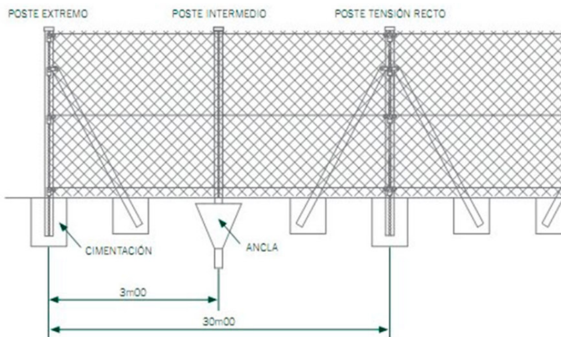
Detalle del montaje de la valla
